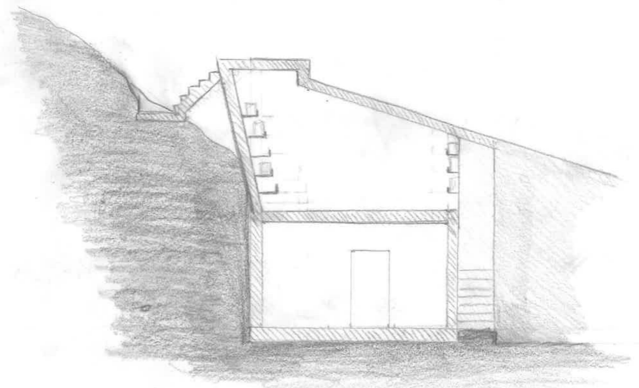
SCHNITT II
