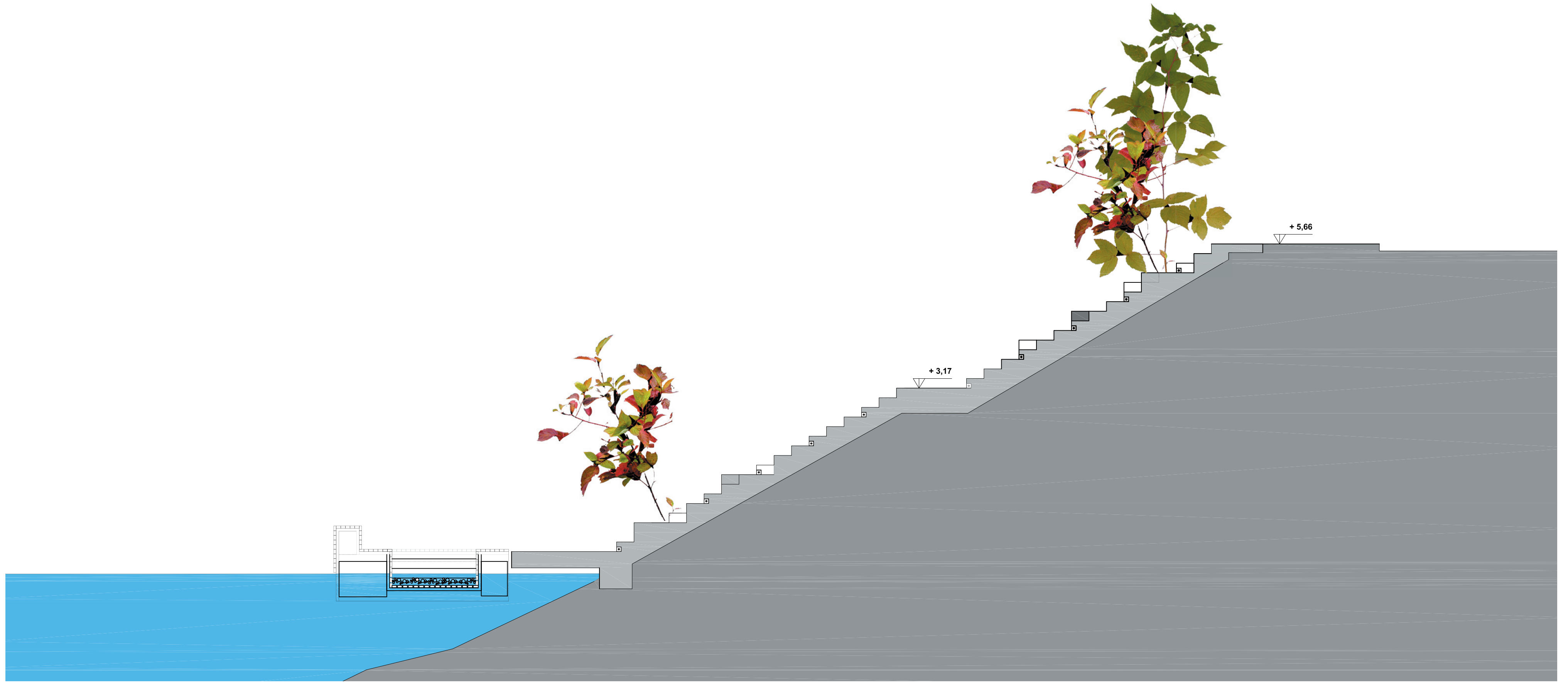
→Schnitt öffentlicher Bereich 1:50
