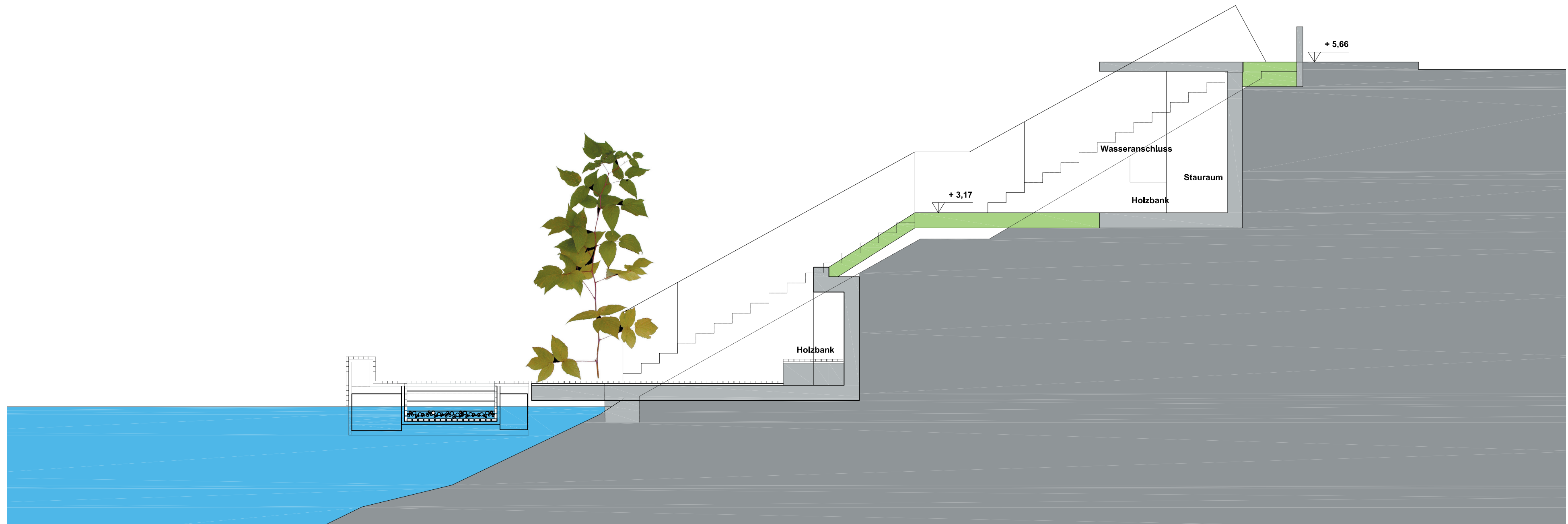
→Schnitt privater Bereich 1:50
