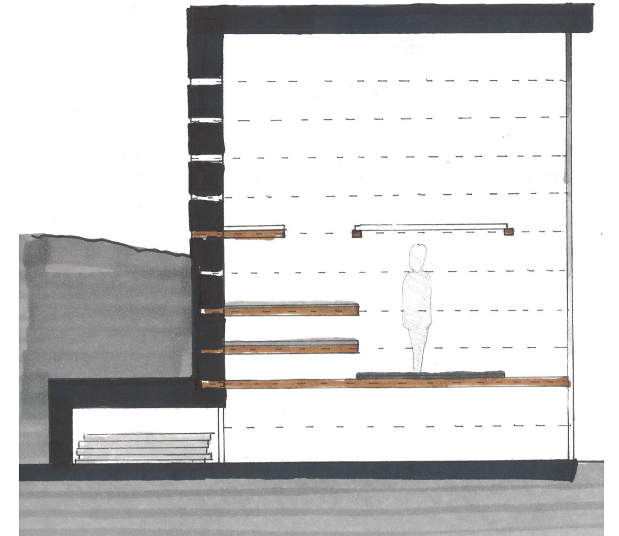
Schnitt M 1:50
